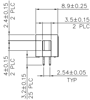
SECTION A-A 1:1
