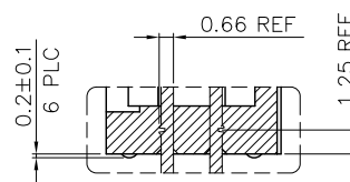
DETAIL B 2:1
