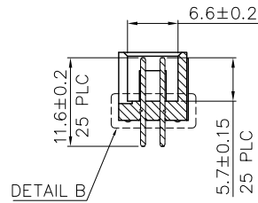
SECTION A-A 1:1
