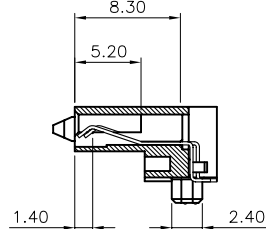
SECTION B-B 1:1
