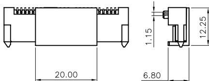
CAP TYPE 2:1
